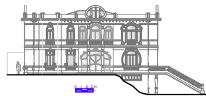
Elevação 01
