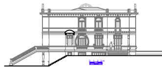
Elevação 03
