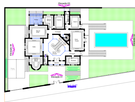
Térreo A = 239,29 m 2
